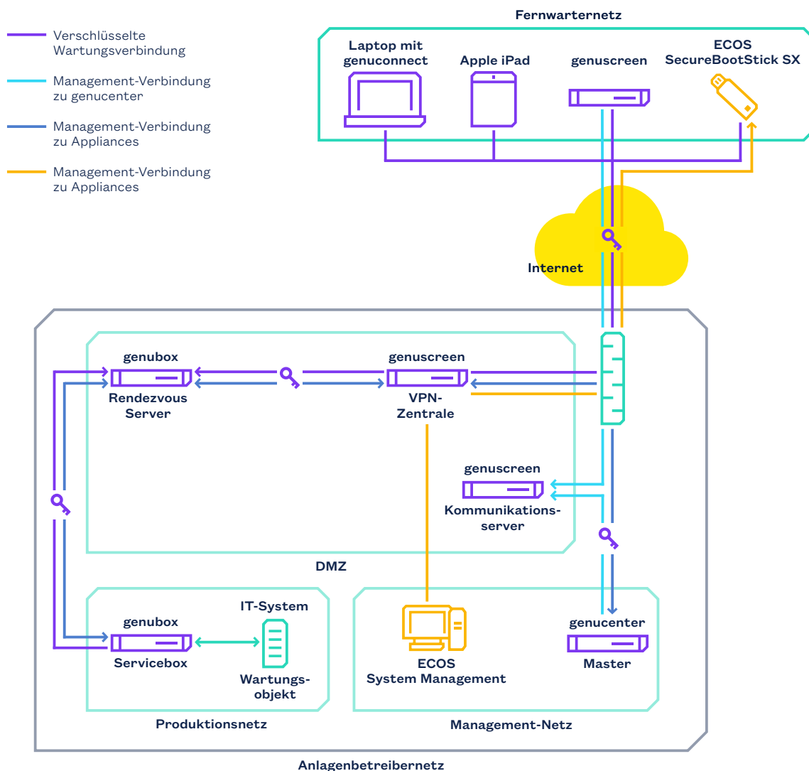
Überblick: Komponenten und Verbindungen bei Fernwartung in ein VS-NfD-Netz
