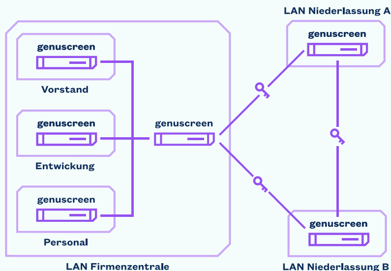
Sicherheitszonen und verschlüsselte Datenkommunikation mit genuscreen
