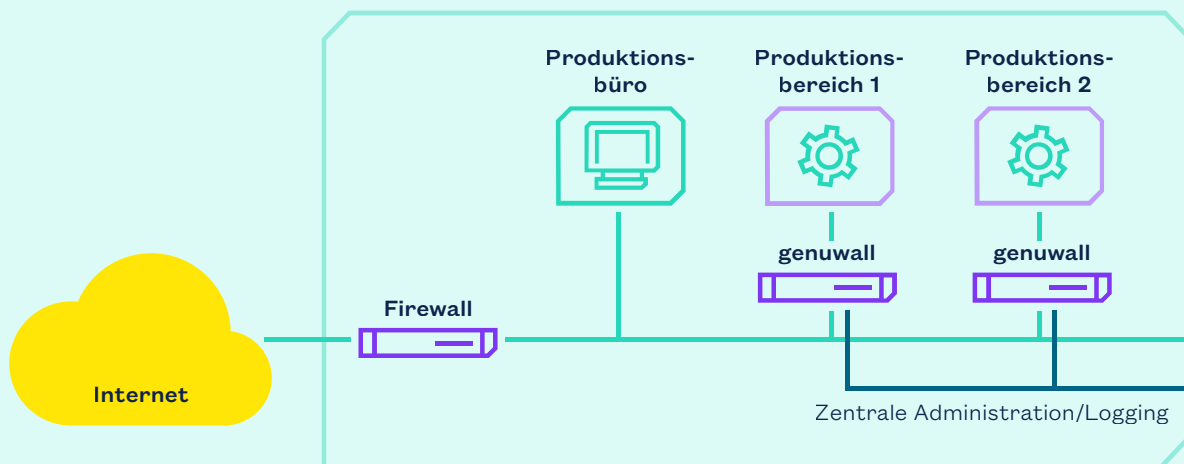
Zonenbildung für sichere Produktionsbereiche mit genuwall
